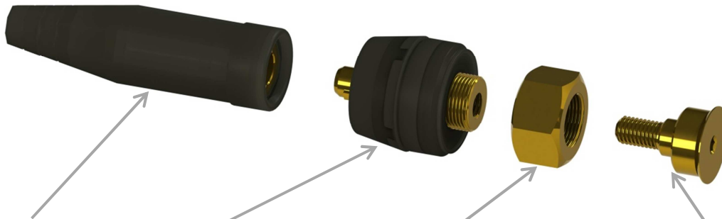
Schweißkabelbuchse (Artikelnr. 000810.3)
